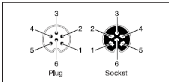
图 40.2: DCN 插头和插座，连接
