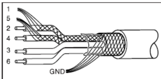
图 40.3: DCN 电缆，连接
